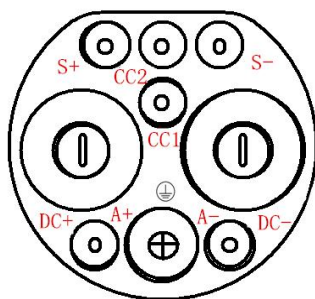
图 1-2 充电插头接口图
