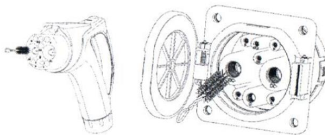
图 3-10 清洁充电枪及插座
