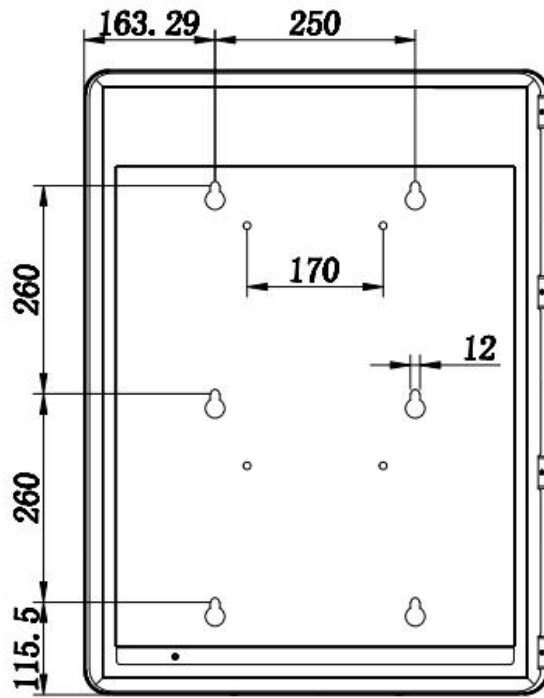
壁挂安装正视图
